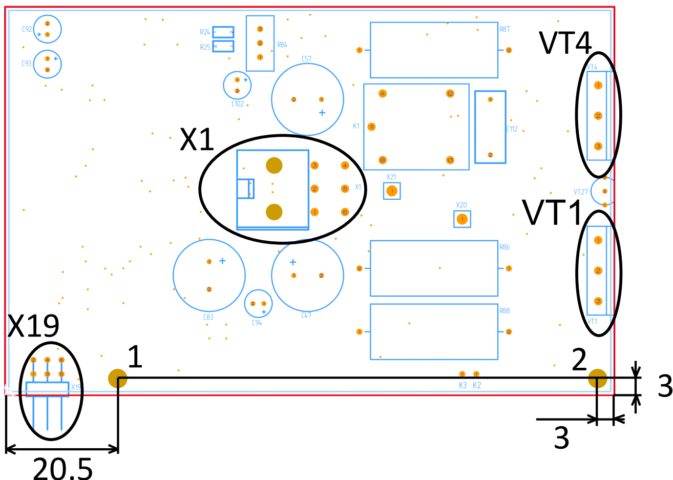
Плата усилителя мощности Amati Solo AS 4330I v1.1 (вид сверху)
